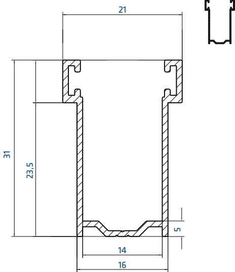
Код направляющей 36764 (на замену) 31x16x31
