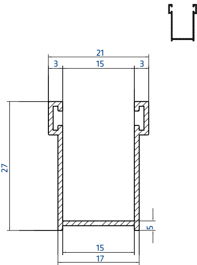
Код направляющей 919 (на замену) 28x17x28 мм
